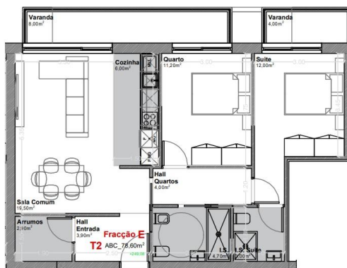
Planta da Fracção
