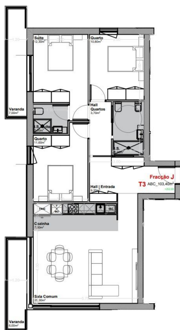
Planta da Fracção
