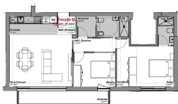
Planta da Fracção
