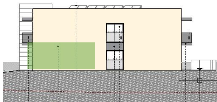
Alçado Lateral
