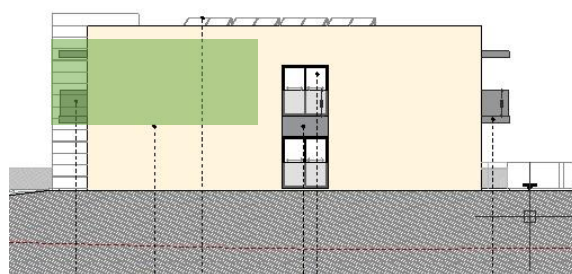
Alçado Lateral
